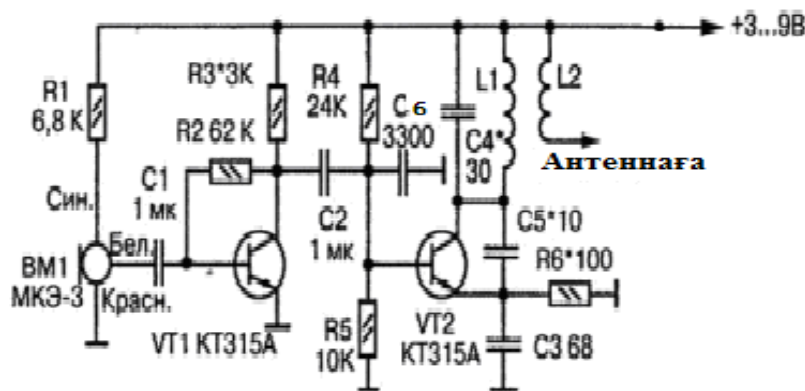
2-мысал. Осы стендпен күнделікті тұрмыс қажетінде қолданылатын қарапайым радиомикрофонды жасау қажет болсын (6-сурет). Радиомикрофон екі транзисторлы схема бойынша құрылған. Транзистор VT1 микрофоннан (BM1) электр тербелістері түрінде келетін дыбыс сигналын күшейтуге арналған. Күшейтілген сигнал оның коллекторлық жүктемесінен (R3) конденсатор C2 арқылы келесі транзистордың VT2 базалық электродына тасымалданады. Осы транзистордың коллекторлық тізбегіне C4 және L1 элементтерінен құрылған тербелмелі контур қосылған, яғни бұл транзистор жоғары жиілікті генератордың міндетін атқарады. Дыбыс сигналы осы тербелістерді жиілігі бойынша модуляциялайды.
