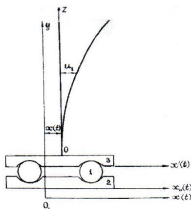
Сурет 2. Қозғалмалы табанды теңселмелі тіректегі серпімді дене тербелісінің схемасы
